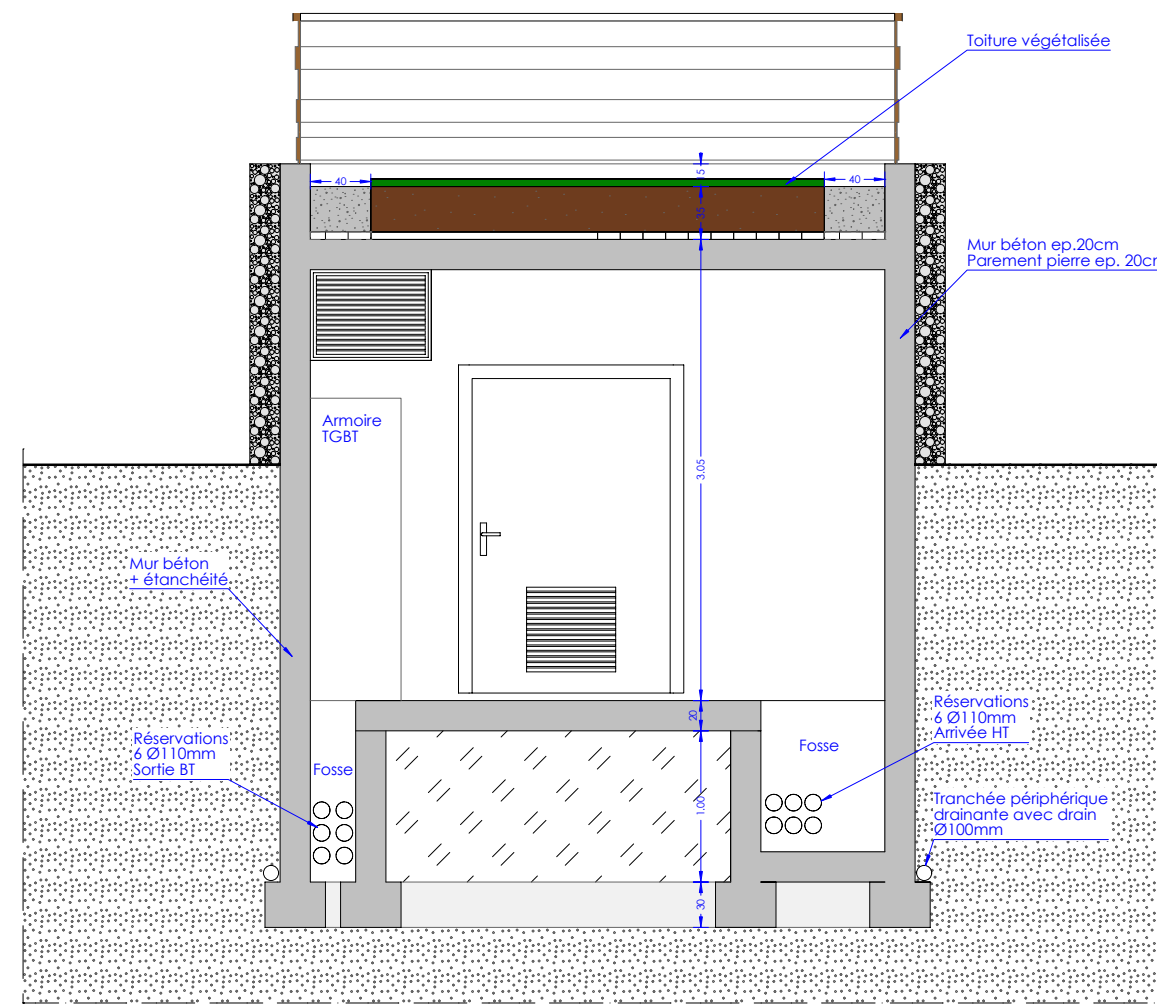
COUPE V-B1
