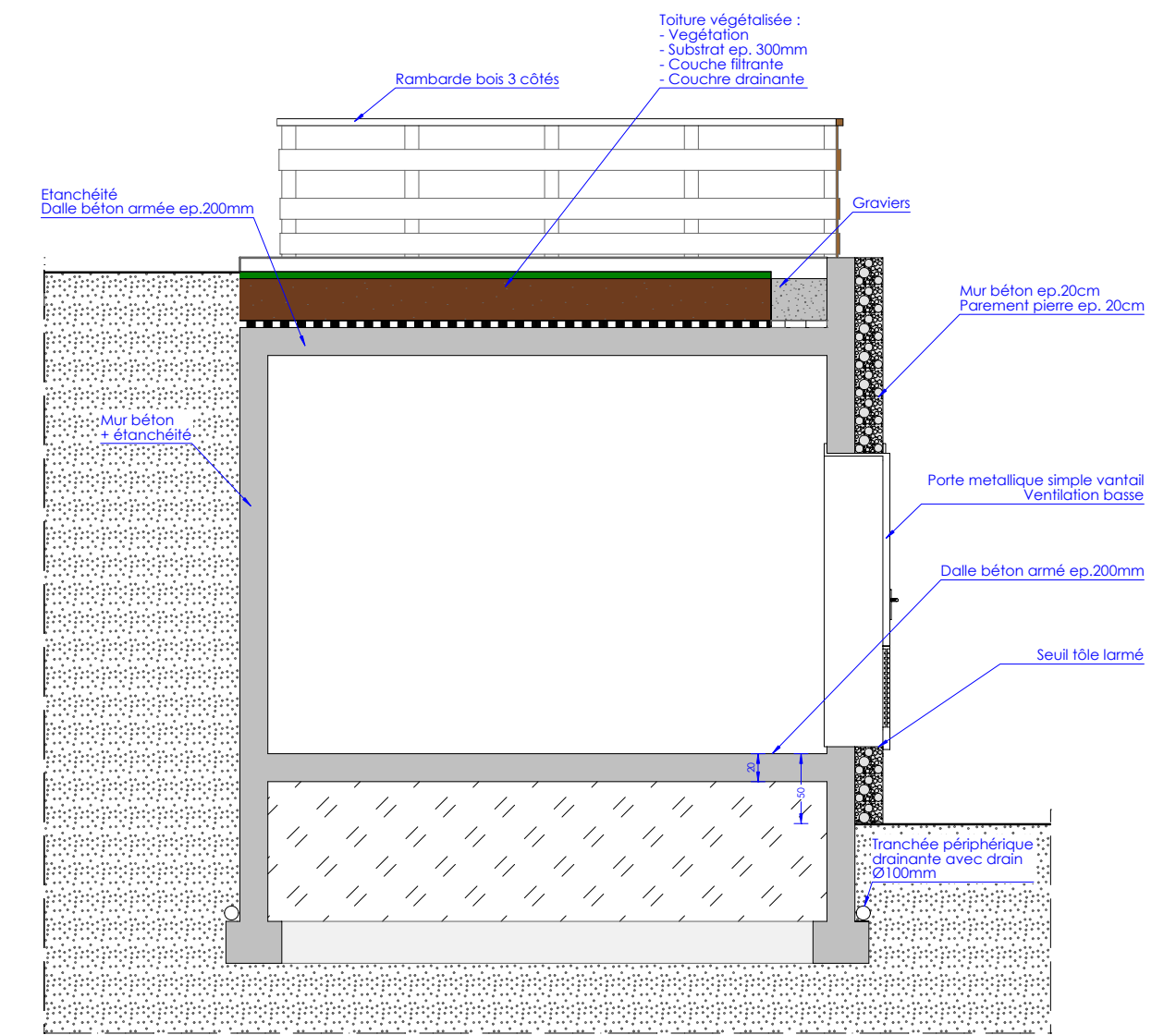
COUPE V_B2
