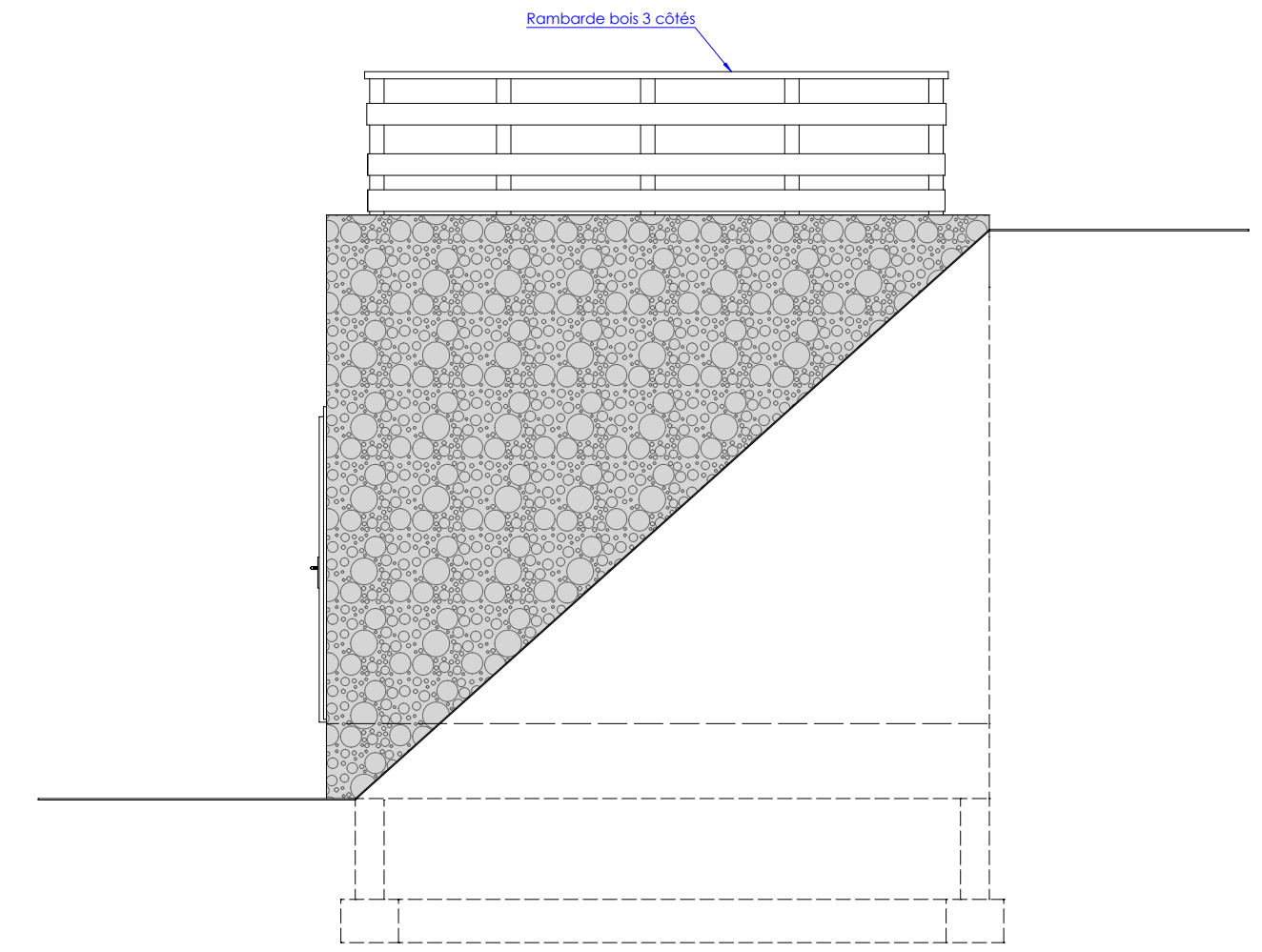
FACADE SUD-EST
