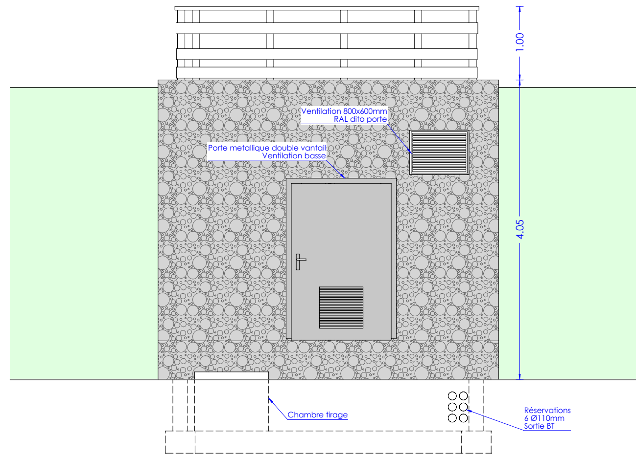
FACADE SUD-OUEST
