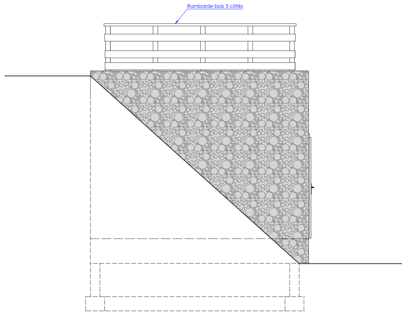
FACADE NORD-OUEST
