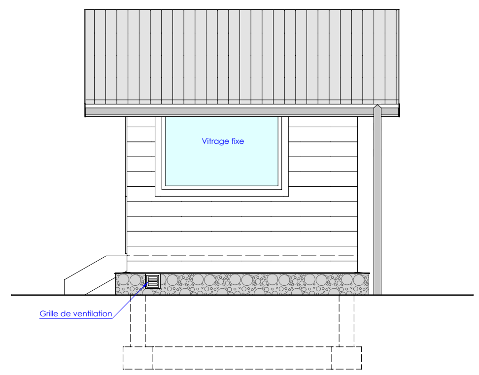
FACADE EST
