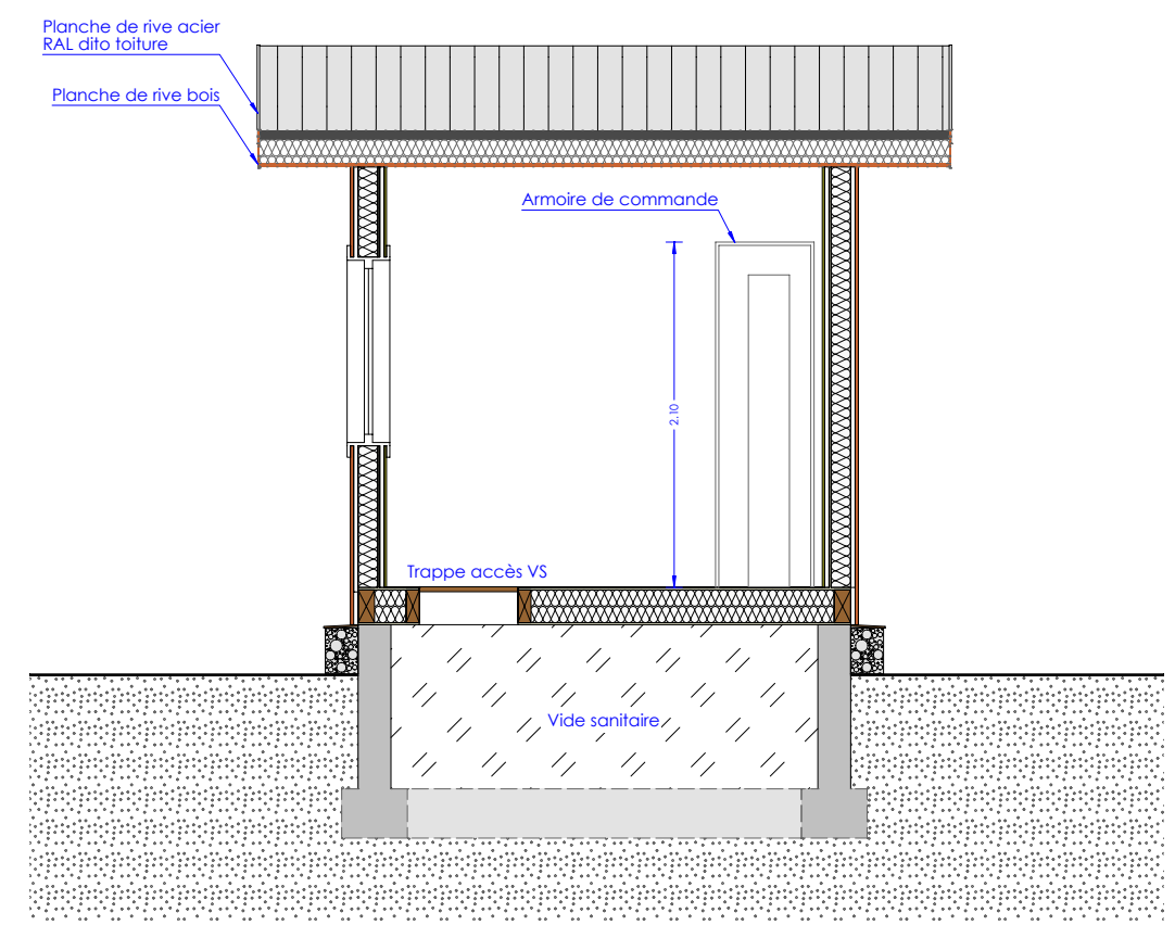
COUPE MP-A2
