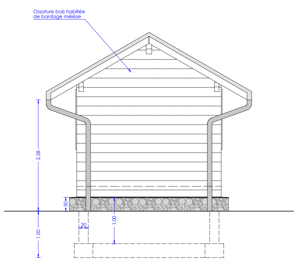
FACADE NORD
