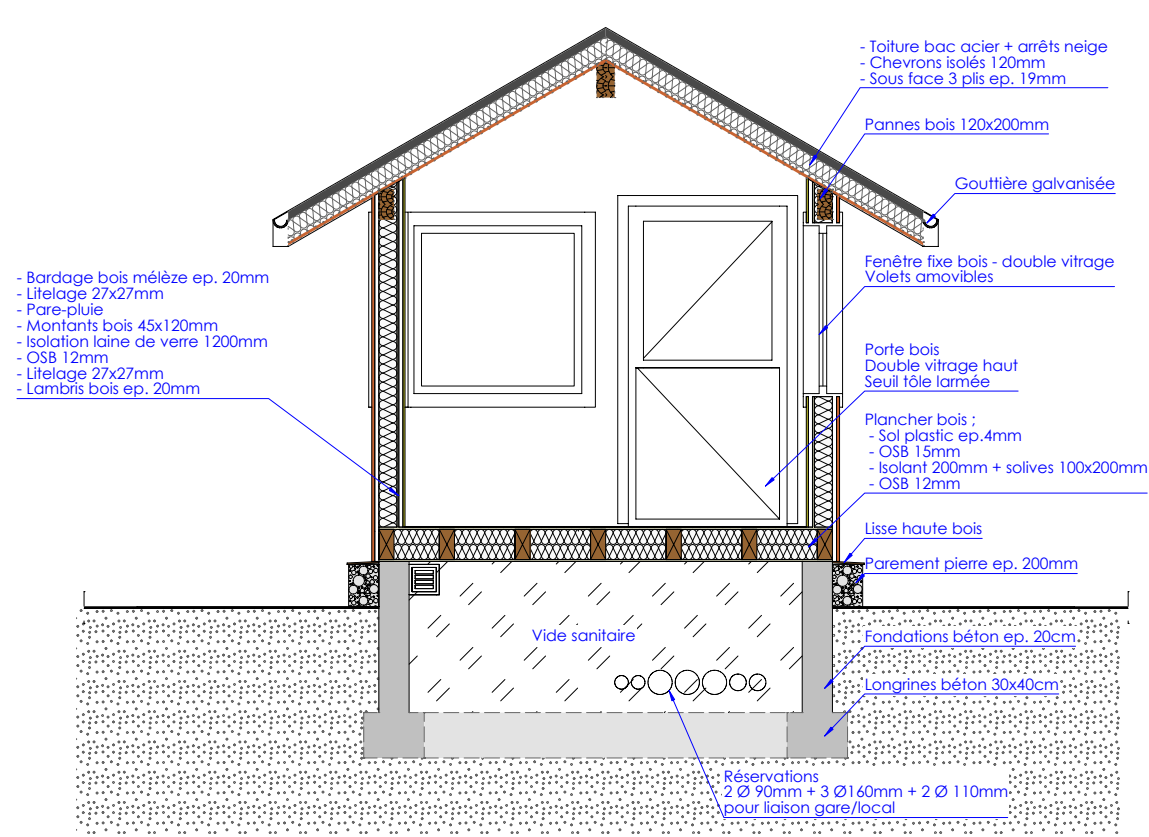
COUPE MP-A1
