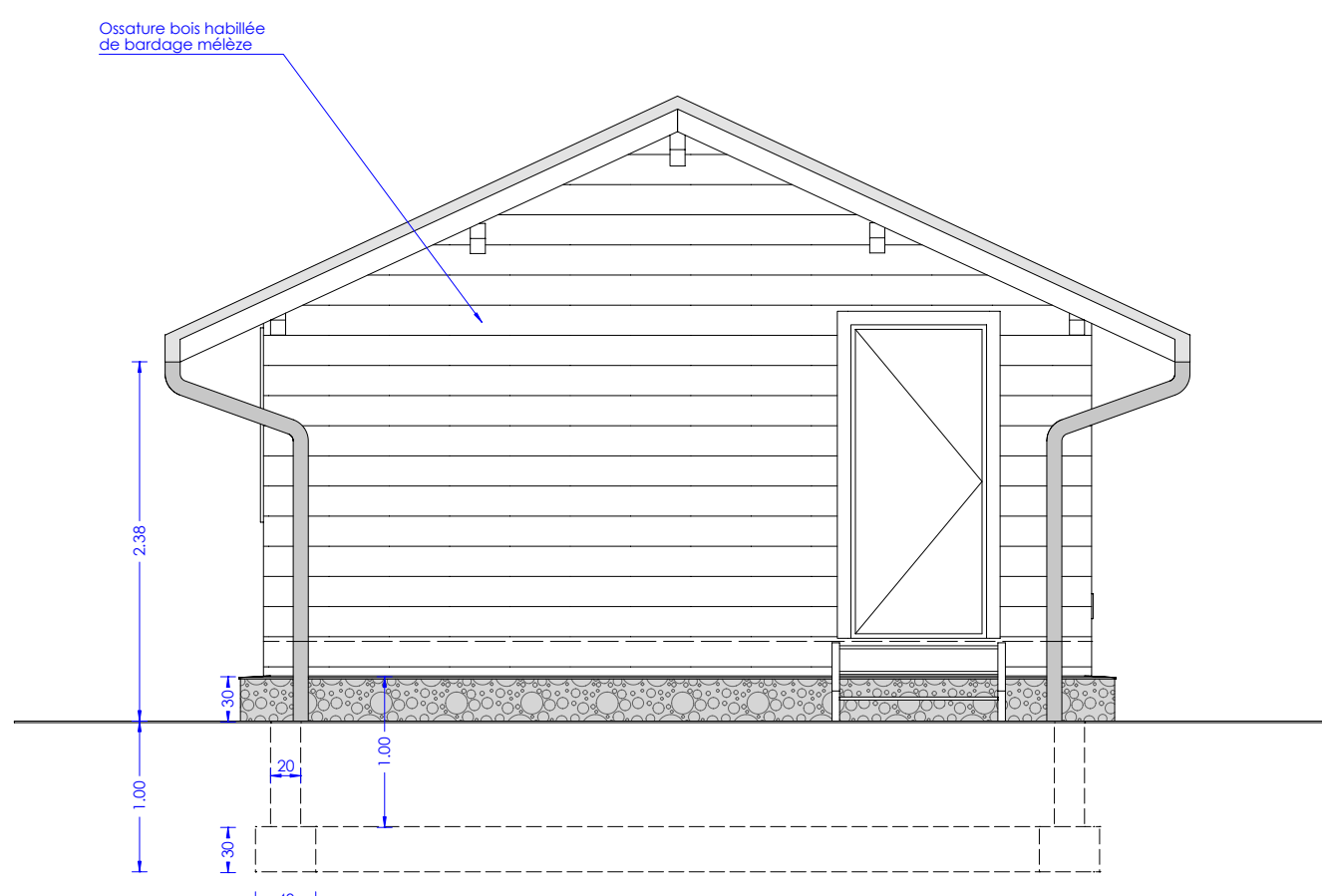
FACADE EST
