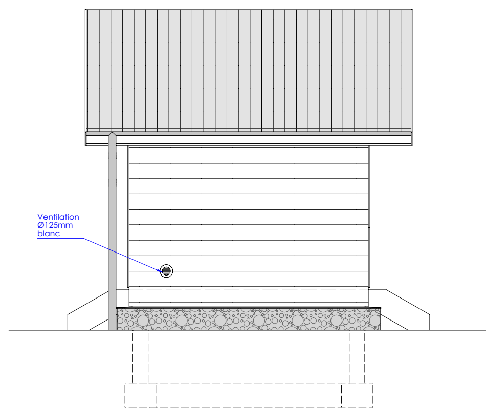
FACADE NORD
