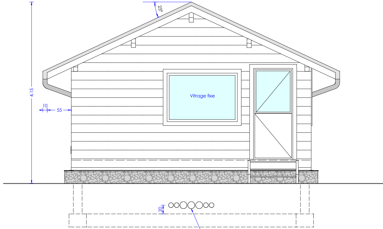
FACADE OUEST
