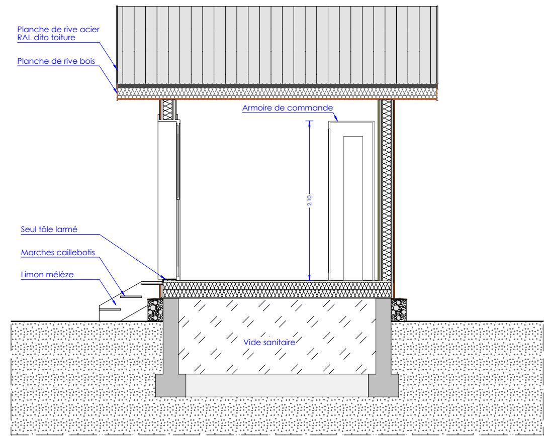
COUPE MP-B2
