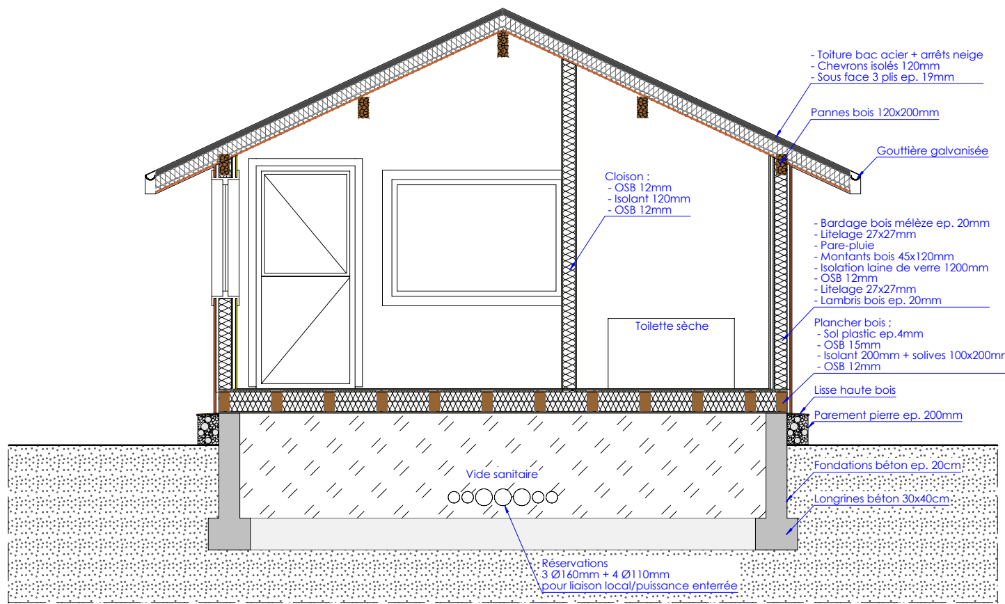
COUPE MP-B1
